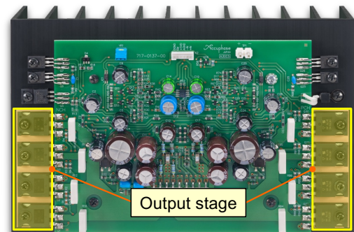
E-700 Power Amplifier Module
